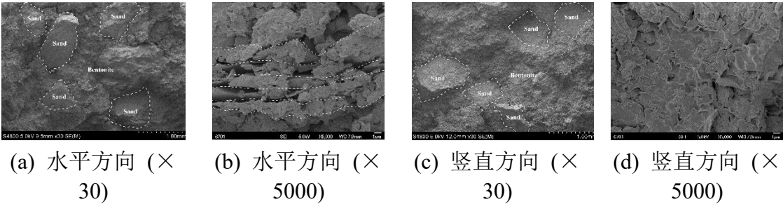
图 2 砌块不同方向扫描电镜图片
