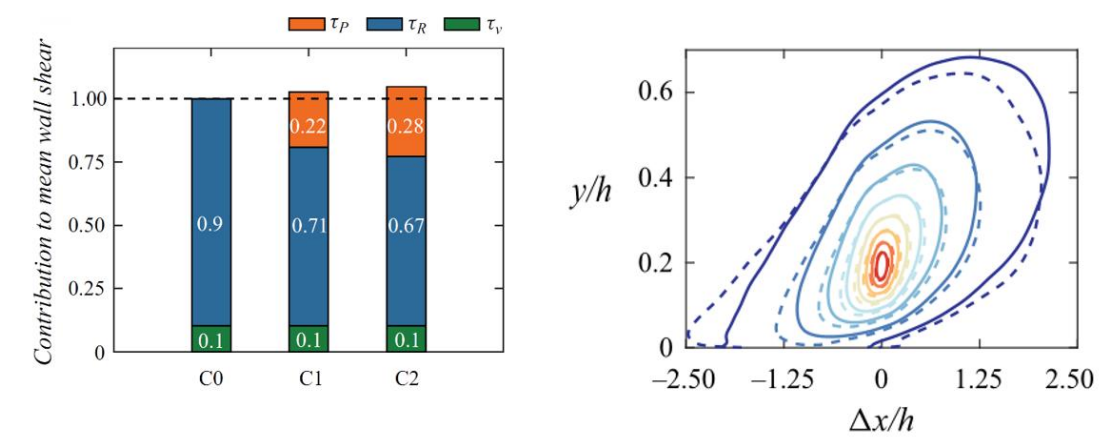
图 1 壁面剪切力 图 2 互相关函数
