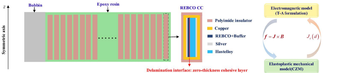
图 1 浸渍超导线圈的二维简化计算模型与引入内聚力本构的电磁-力耦合模型
