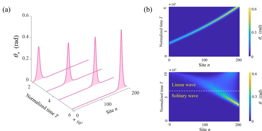
图2 矢量孤子的单向放大和不对称传输
