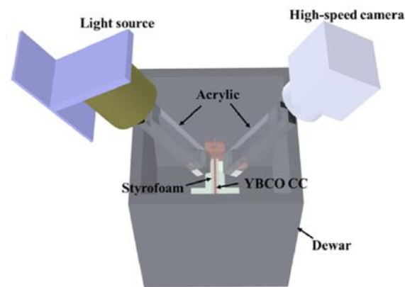
图 1 拍摄装置图
